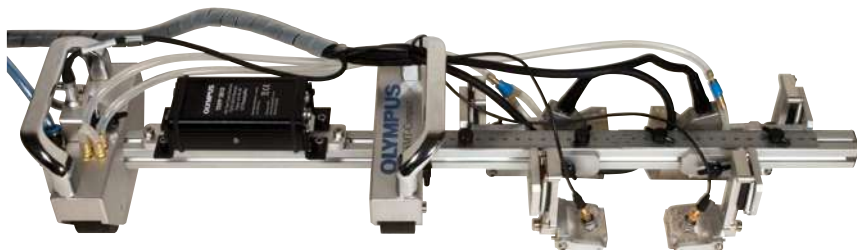
Configuración adecuada para áreas de difícil acceso, como las soldaduras entre tubería y componente.
