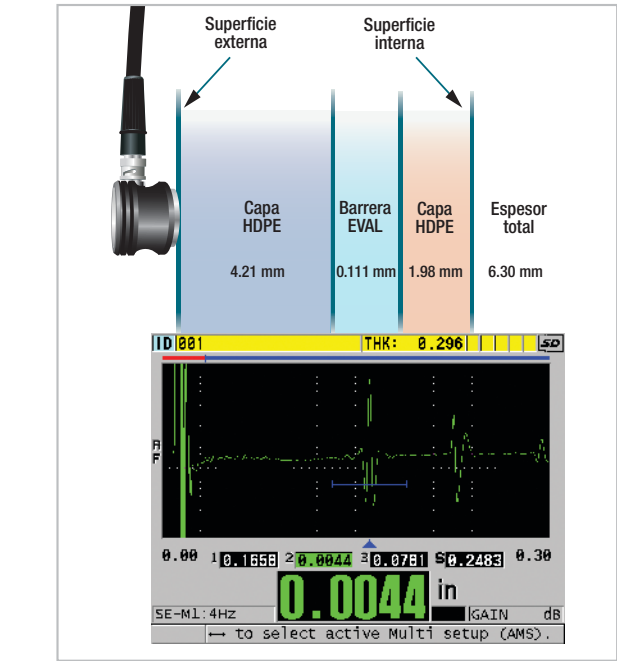
El medidor de espesores 38DL PLUS efectúa simultáneamente la medición precisa de hasta cuatro capas individuales.
