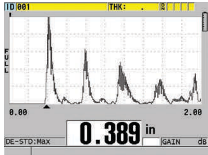
Parámetro de pantalla para exteriores en modo A-scan
