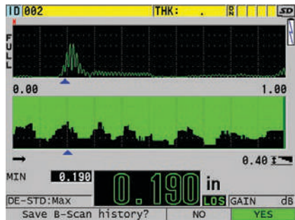
Parámetro de pantalla para exteriores en modo B-scan
